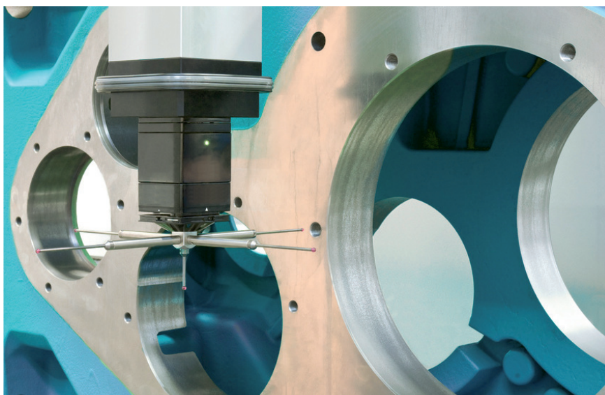
3D-Koordinatenmessung
