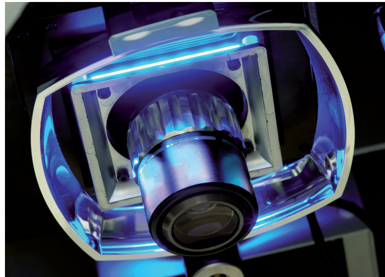
Messobjektiv mit Vierquadranten-Ringlicht
